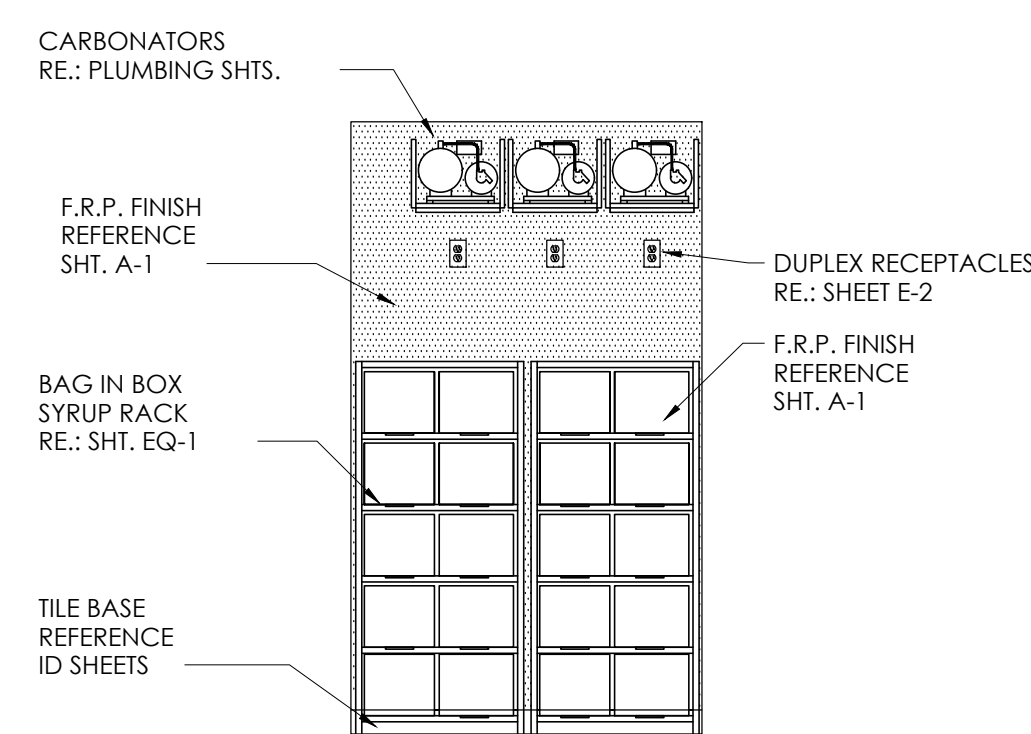
C ELEVATION SCALE: 3/8" = 1'-0"
